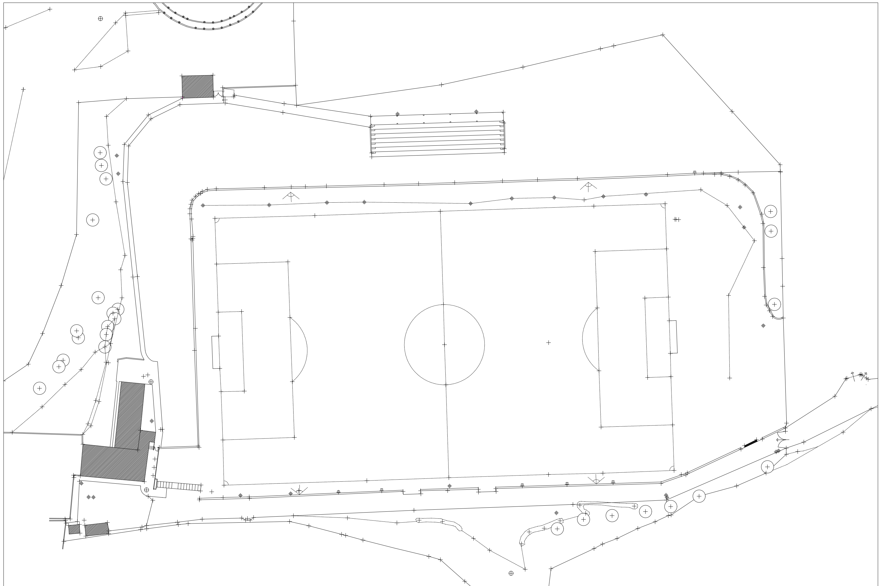
CENTRO SPORTIVE DEL BARRO - PLANIMETRIA GENERALE - SCALA 1:500
